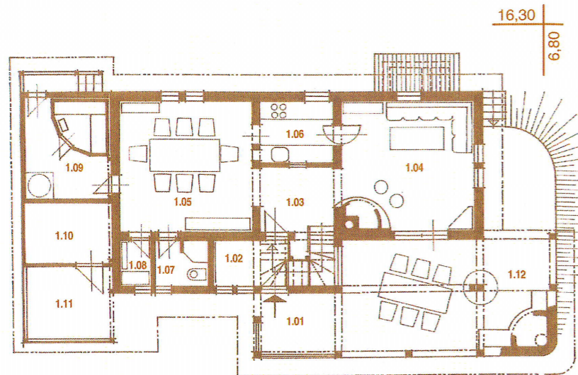
pôdorys prízemia
