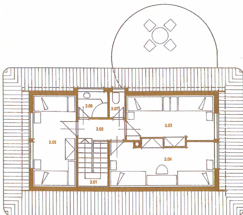
pôdorys podkrovia
