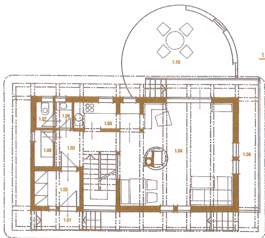
pôdorys prízemia
