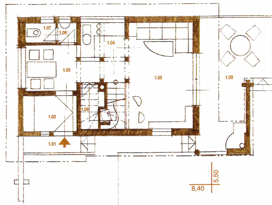
pôdorys prízemia
